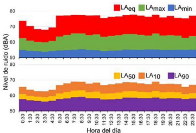
Figura 1. Nivel promedio de ruido a lo largo de un día de muestreo para los parámetros acústicos. Arriba: LAeq, LAmáx y LAmin; abajo: percentiles LA 50 , LA 10 y LA 90 .
