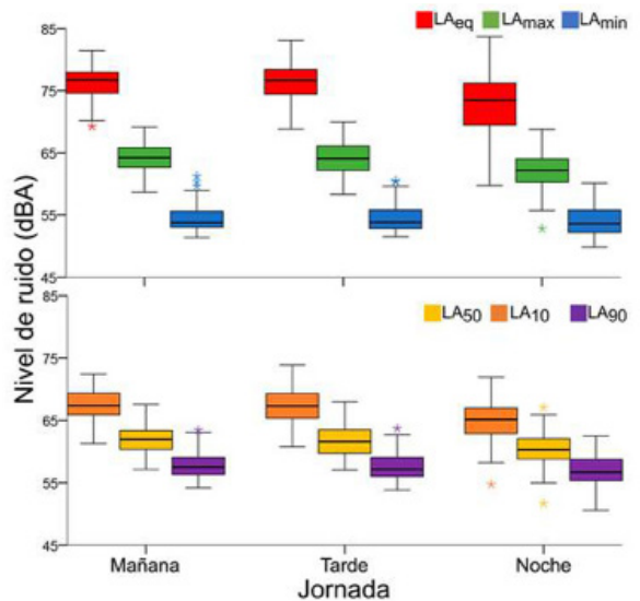
Figura 2. Nivel promedio de ruido por día muestreo para los parámetros (LAeq, LAmáx y LAmin) y los percentiles (LA50, LA10 y LA90) acústicos.
