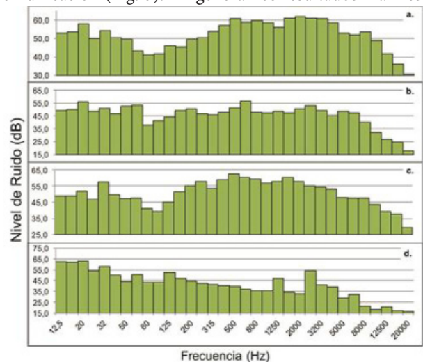
Figura 3. Espectro fuentes de ruido estudiadas. Resultados del espectro de a) monitor de signos A1, b) monitor de signos A2, c) monitor de signos A3, d) teléfono.
